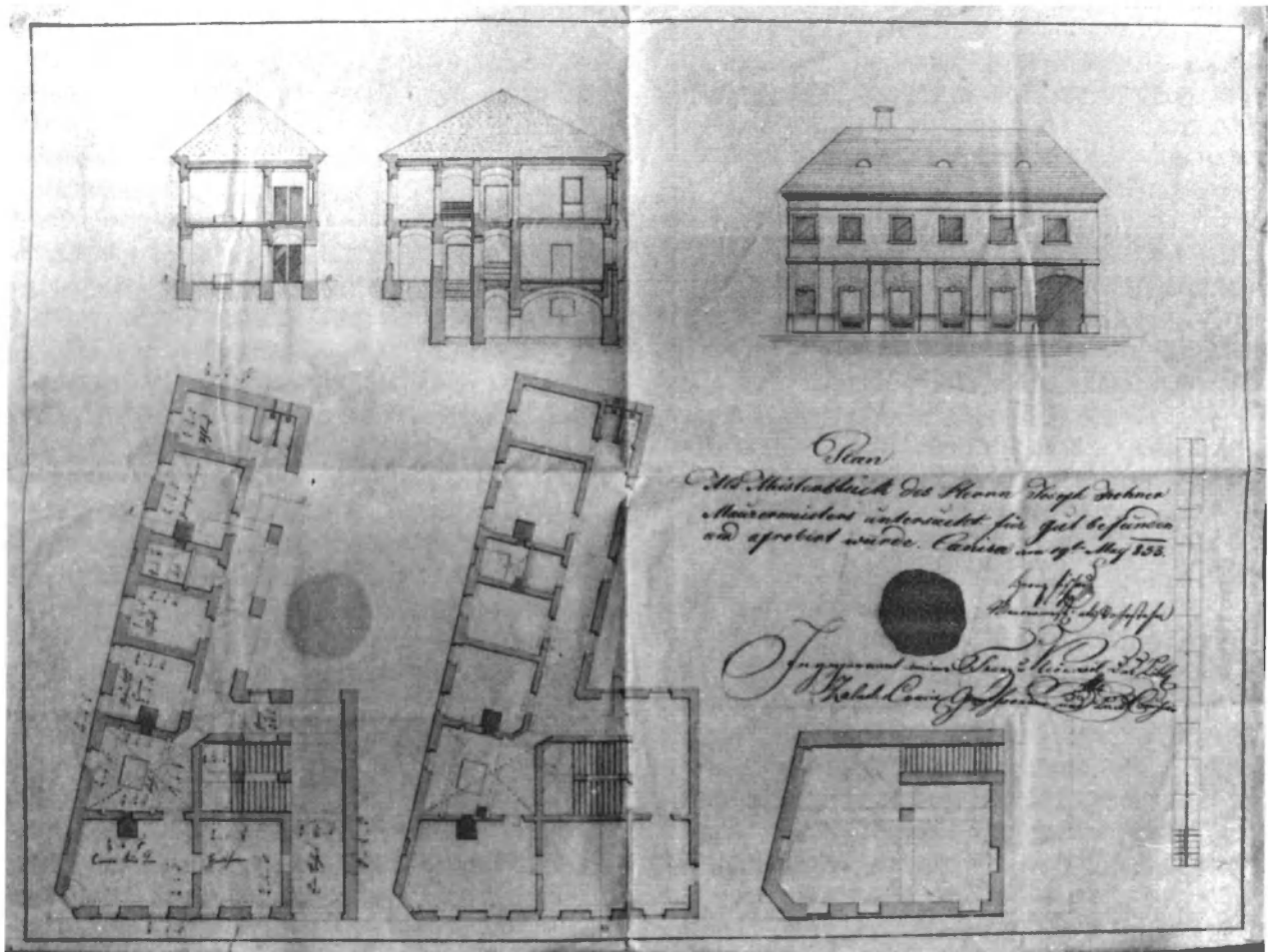
7. kép. Joseph Frohner kőműves remekműként 1833-ban készített tervrajza. (TGYM 72.65.1.)
